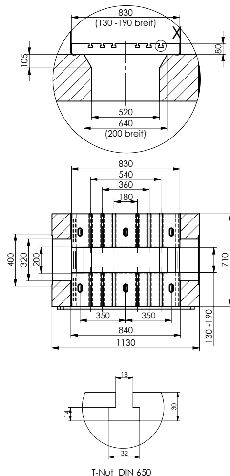
T-Nut DIN 650
